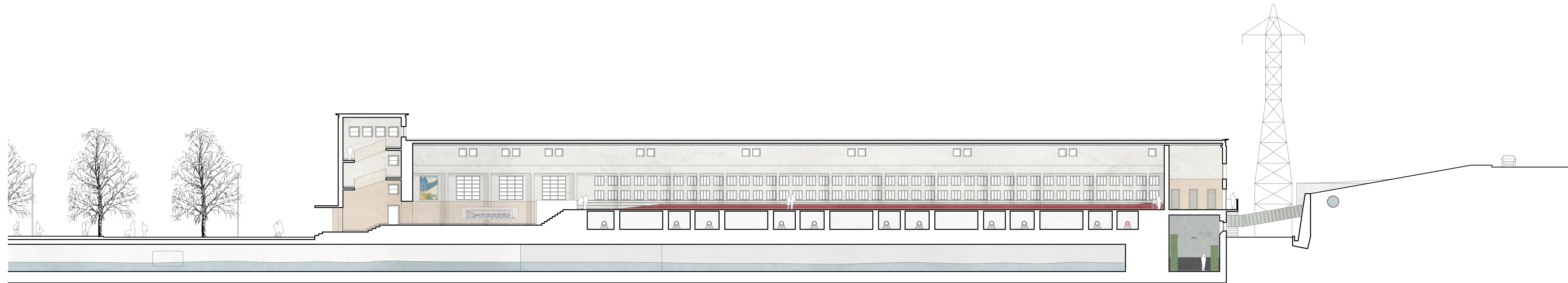
Coupe longitudinale E.E 1.200
