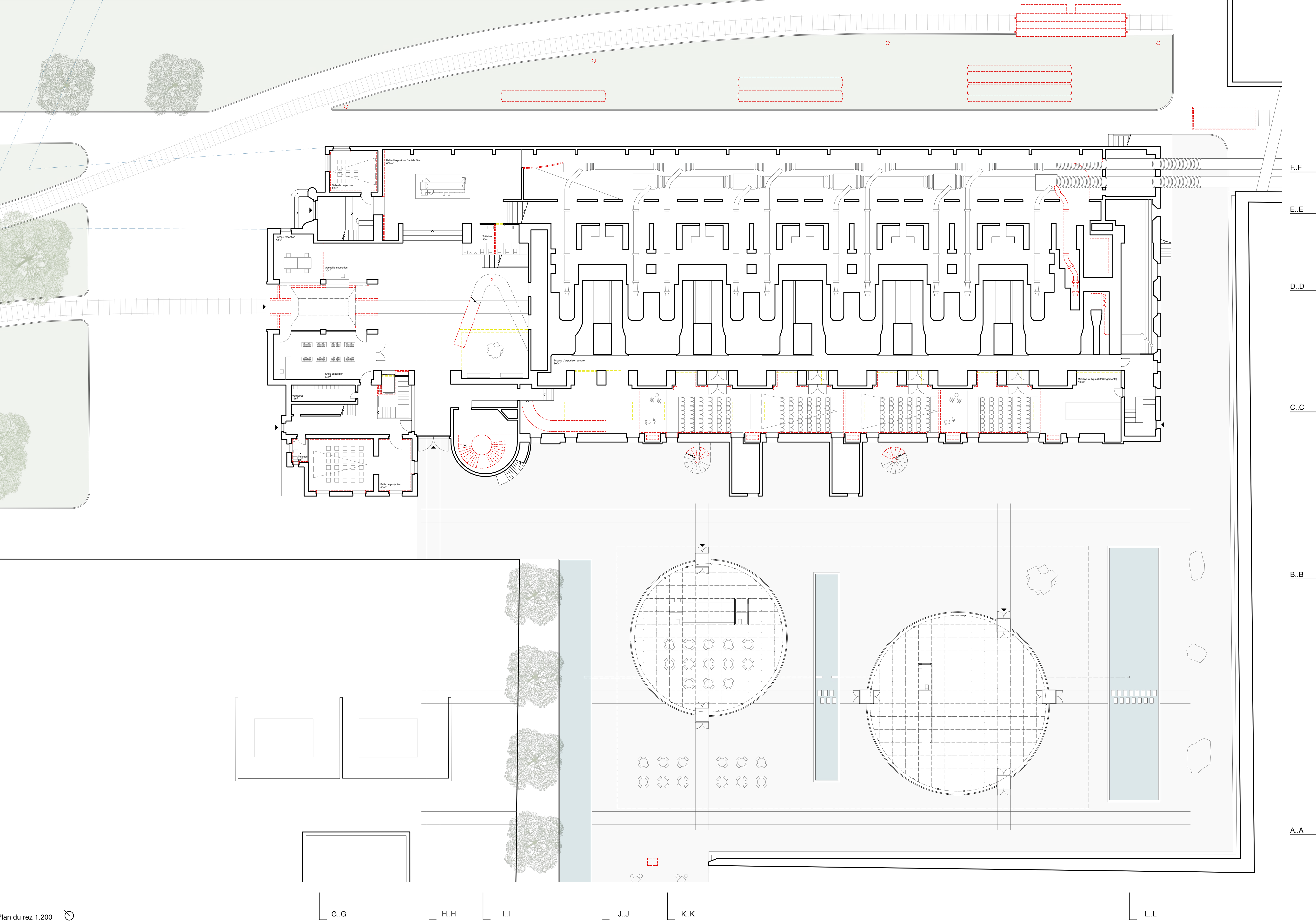
Plan du rez 1.200
