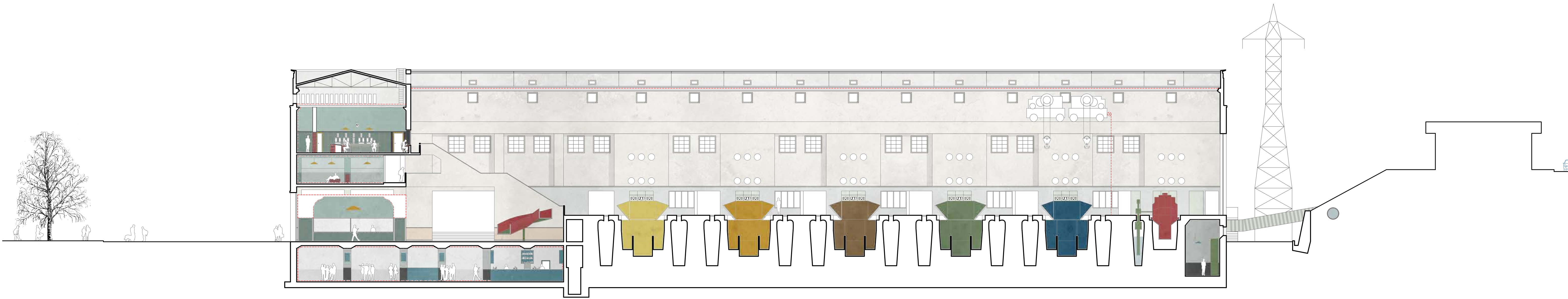
Coupe longitudinale D.D 1.200
