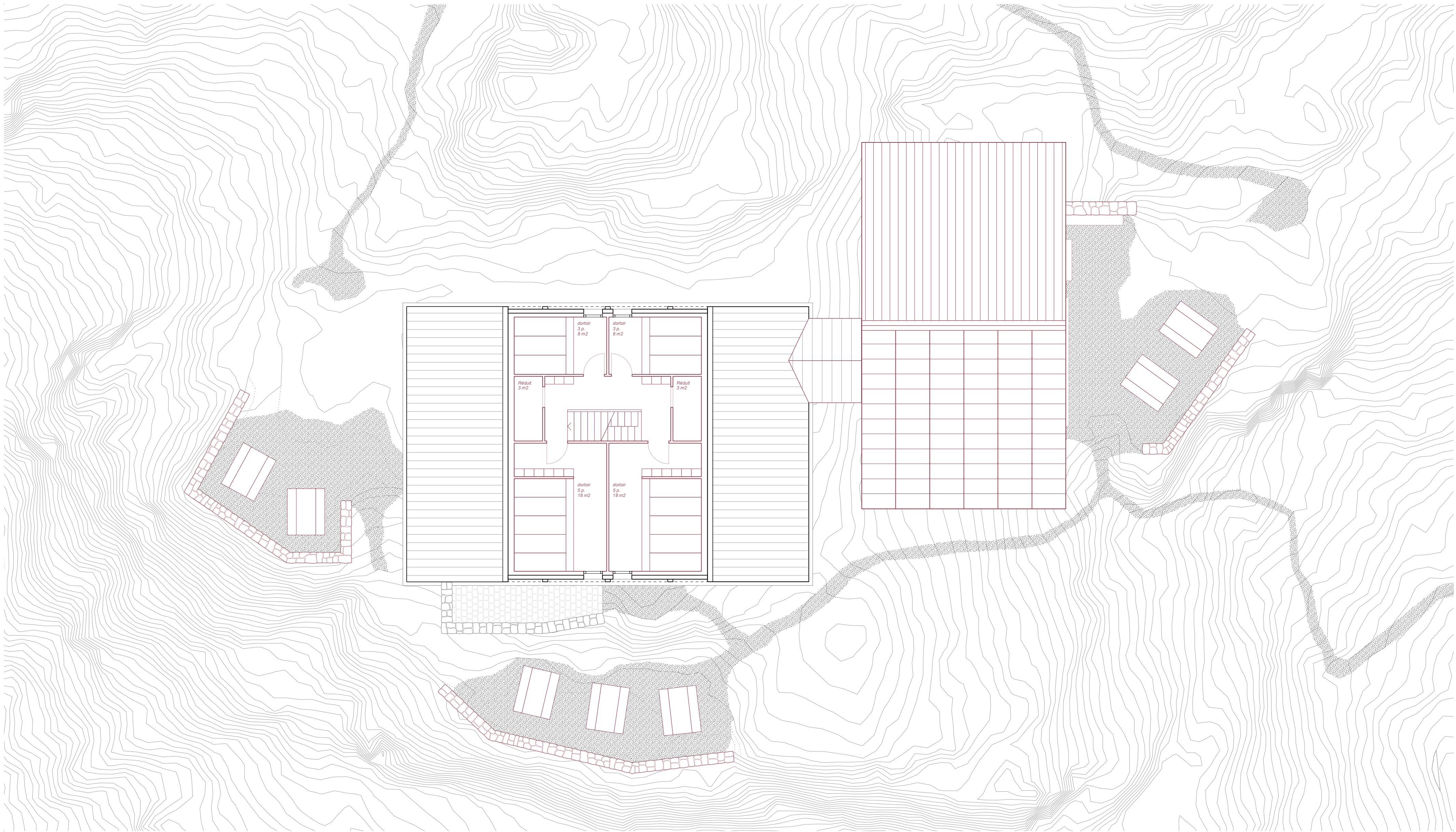
5. Deuxième étage 1:100
