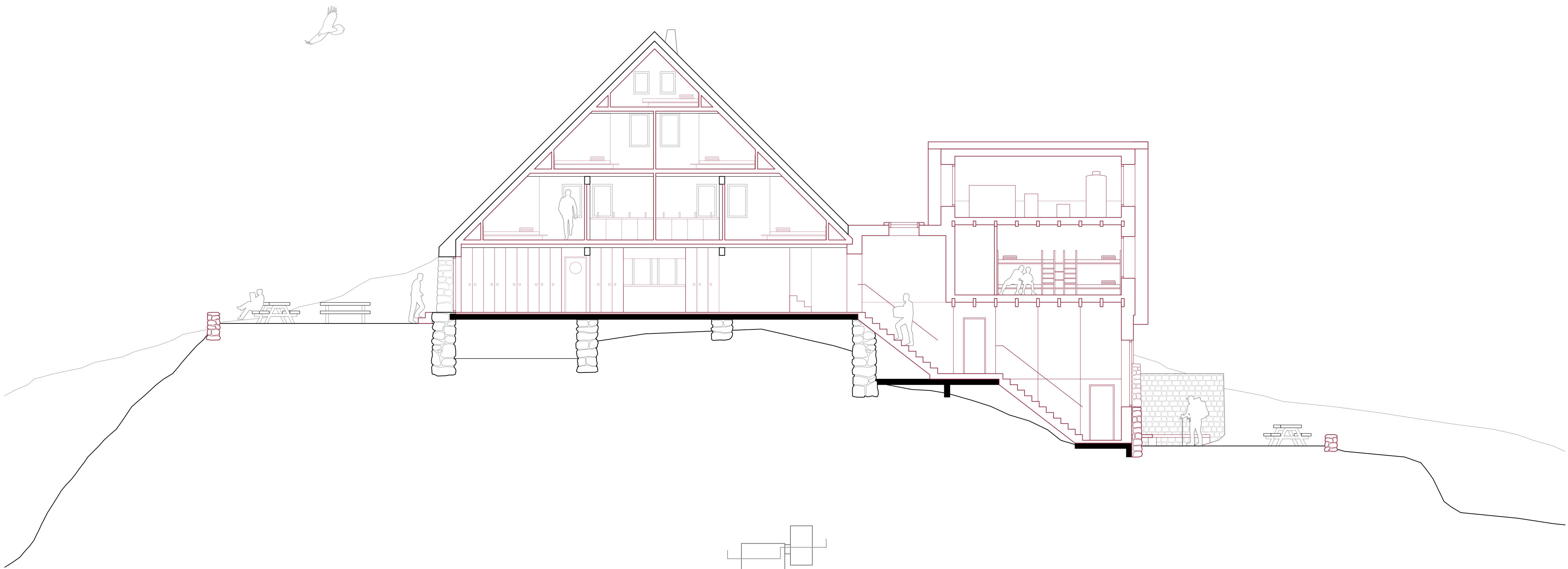
Coupe Est - Ouest 1:100
