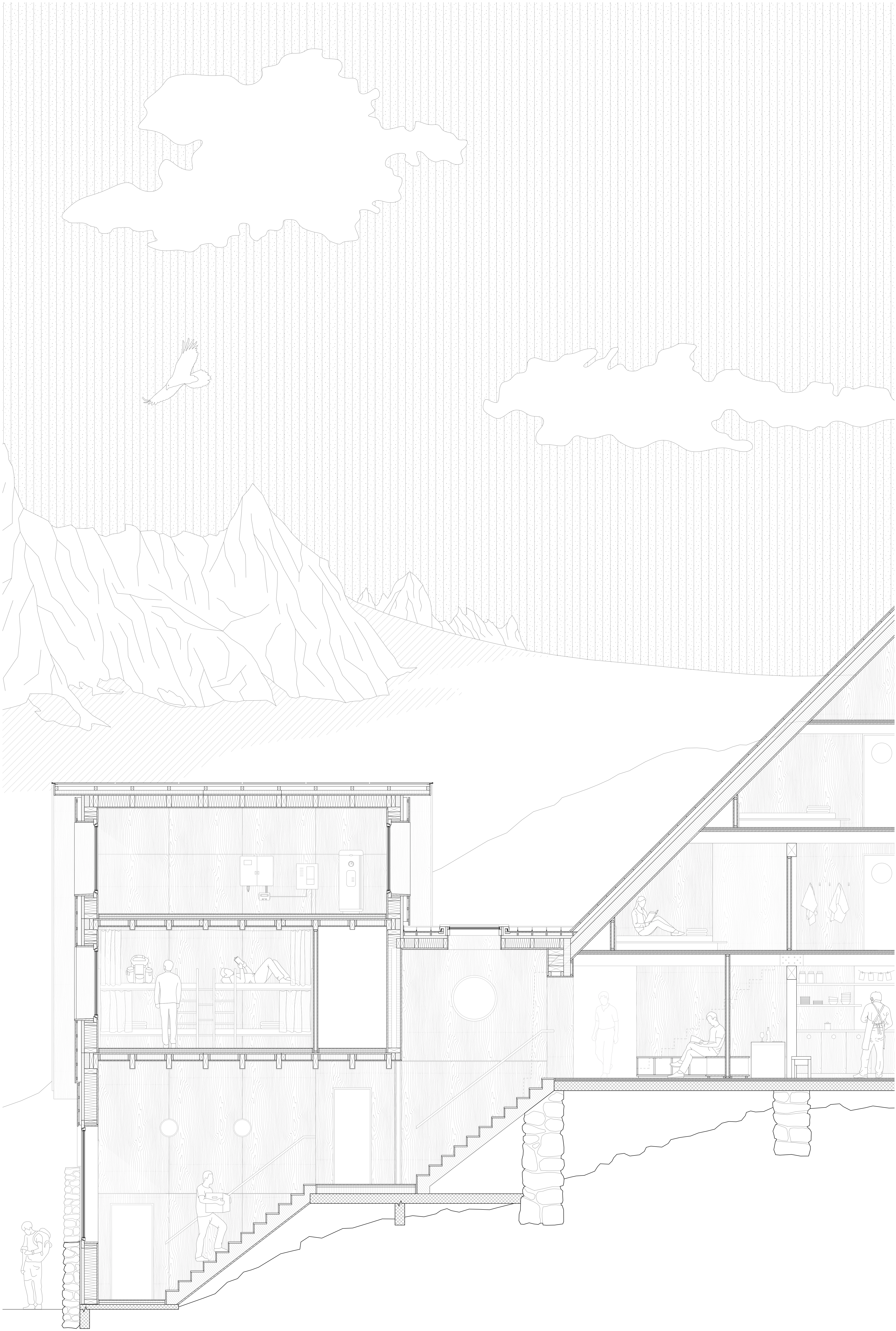
Paliers d'entrée Coupe 1:33
