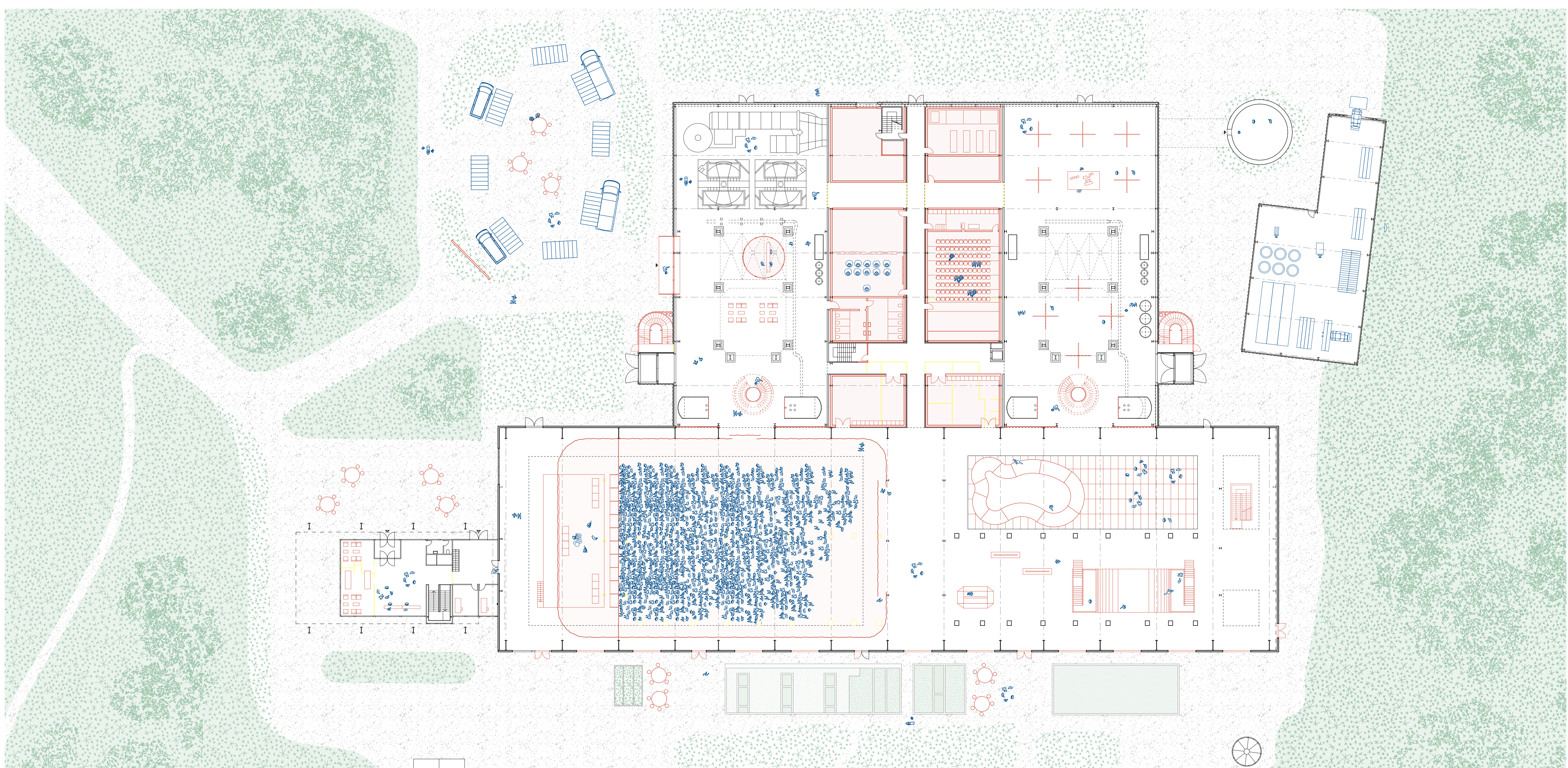
REZ-DE-CHAUSSÉE 1/300
