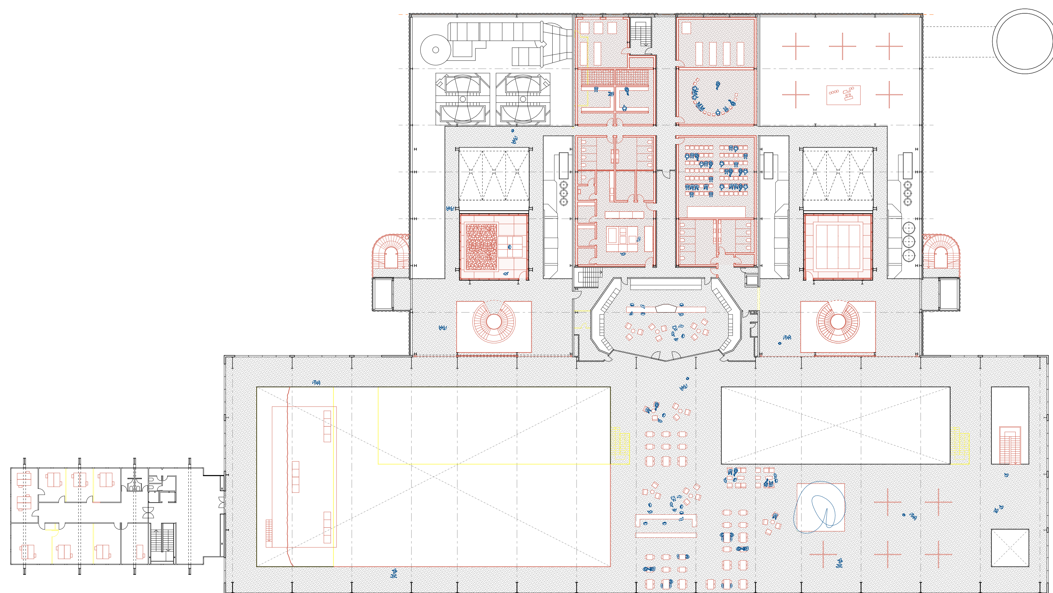
ÉTAGE + 9.00 1/300
