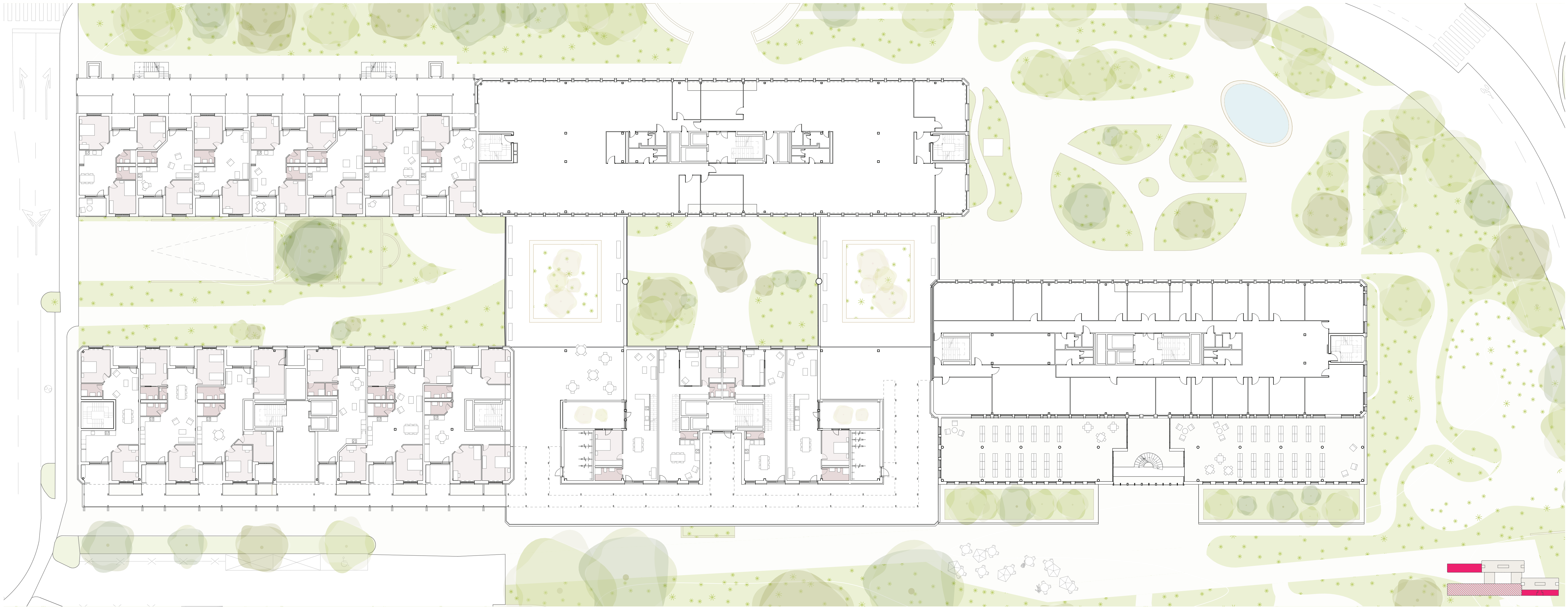
Plan du deuxième étage - 1:250
