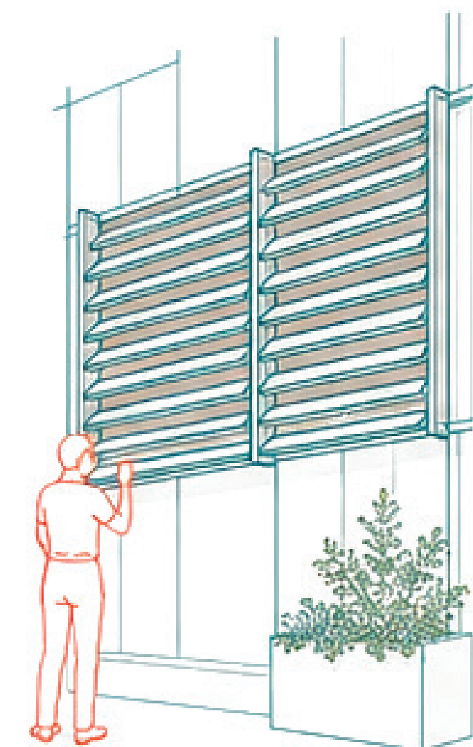
BRISÉ SOLEIL ORIENTABLE
