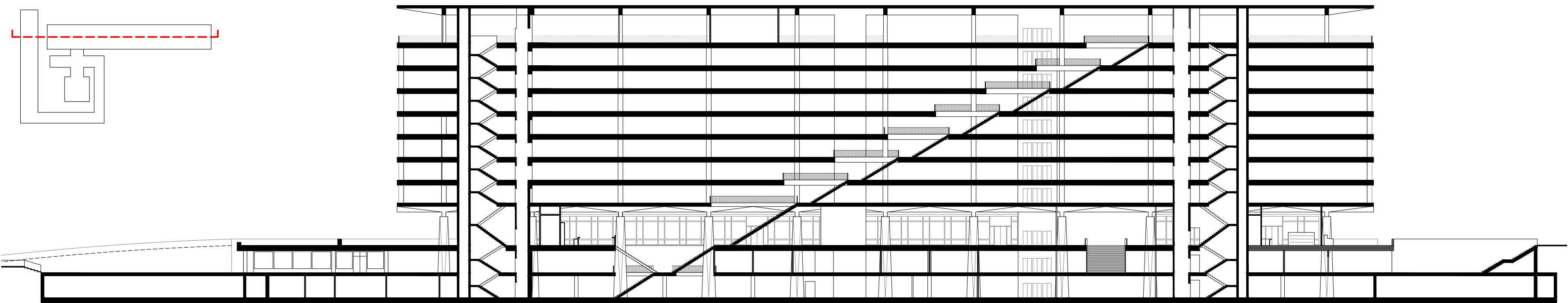
Coupe B_B
